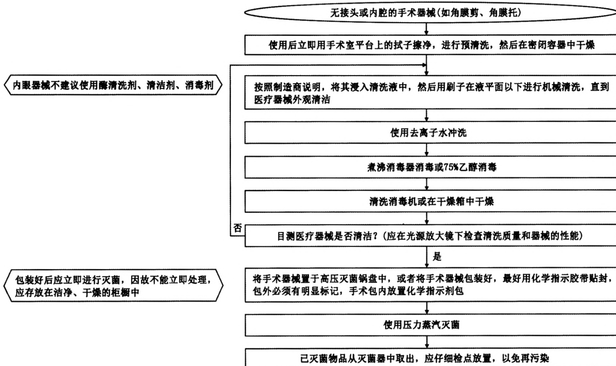
图 11 无接头和内腔的角膜手术器械消毒与灭菌流程
