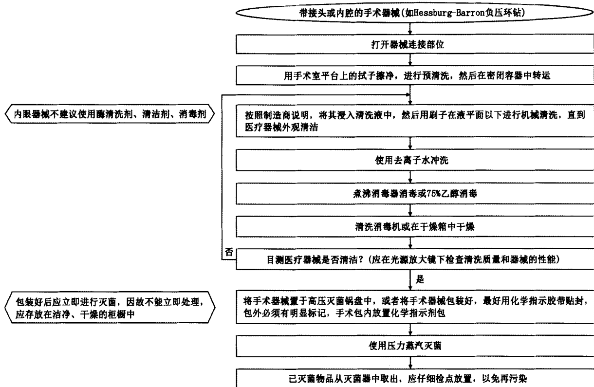
图 14 带接头或内腔的角膜手术器械消毒与灭菌流程
